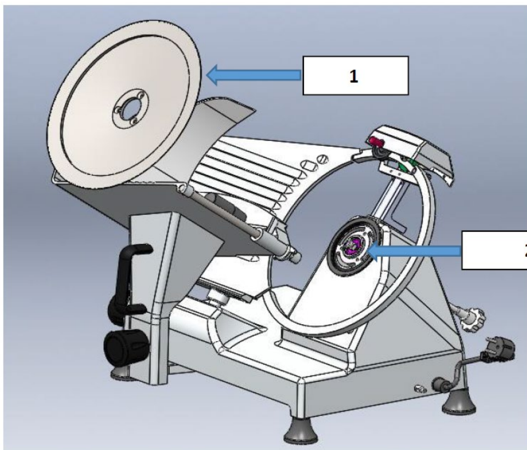
Kuva 2: Kokoanpanovaihe 1 - Asenna terä tuotteelle
