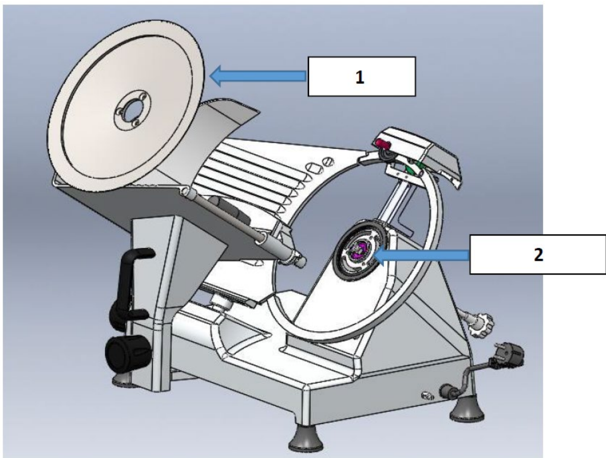
Abbildung 2: Montageschritt 1 - Installieren Sie die Klinge für das Produkt
