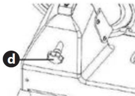
Abbildung 10: Darstellung der Befestigungsschraube (d)
