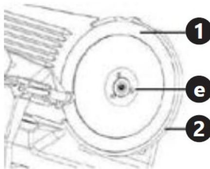
Figur 11: Illustrasjon av justeringsskruer (e), kniv (1) og knivbeskyttelsesring (2)
